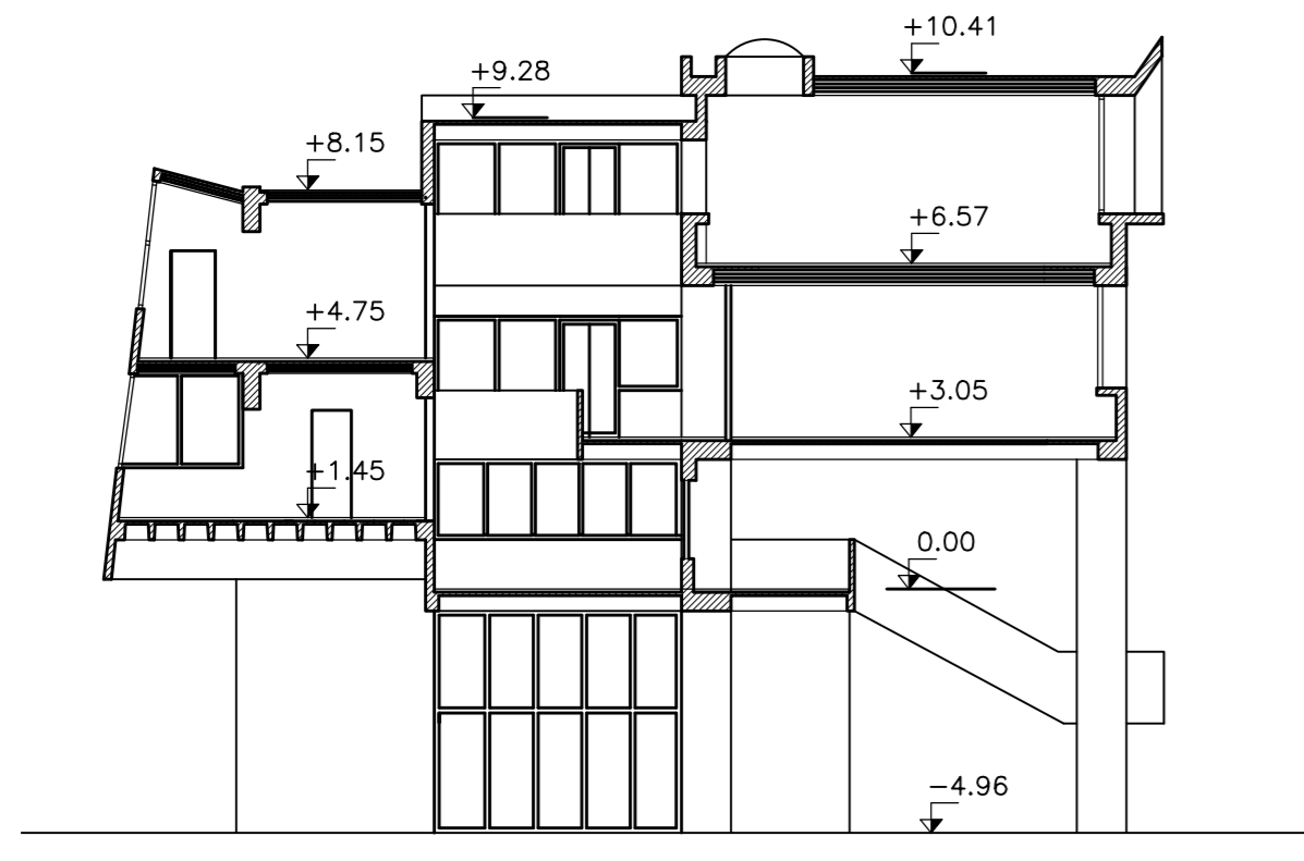
SEZIONE TIPO
