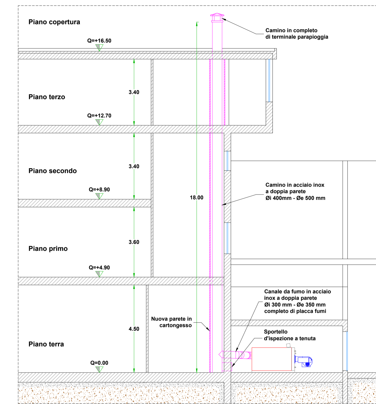
SEZIONE A-A
